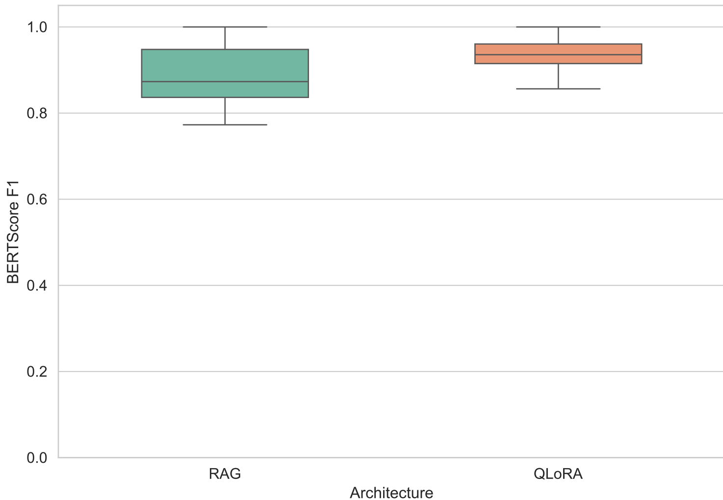
Distribution of Semantic Similarity (BERTScore F1)
