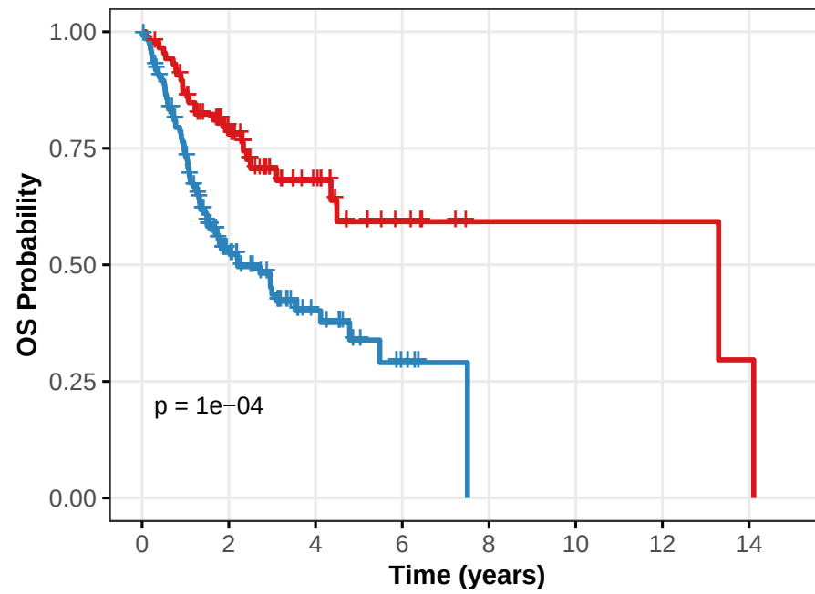
TOPBP1
