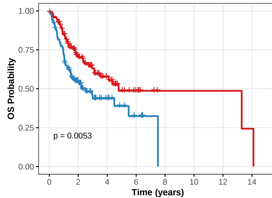
PARP1
