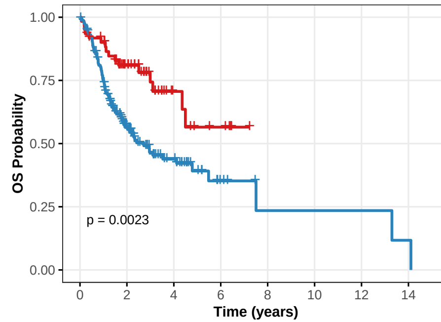
EGFR
