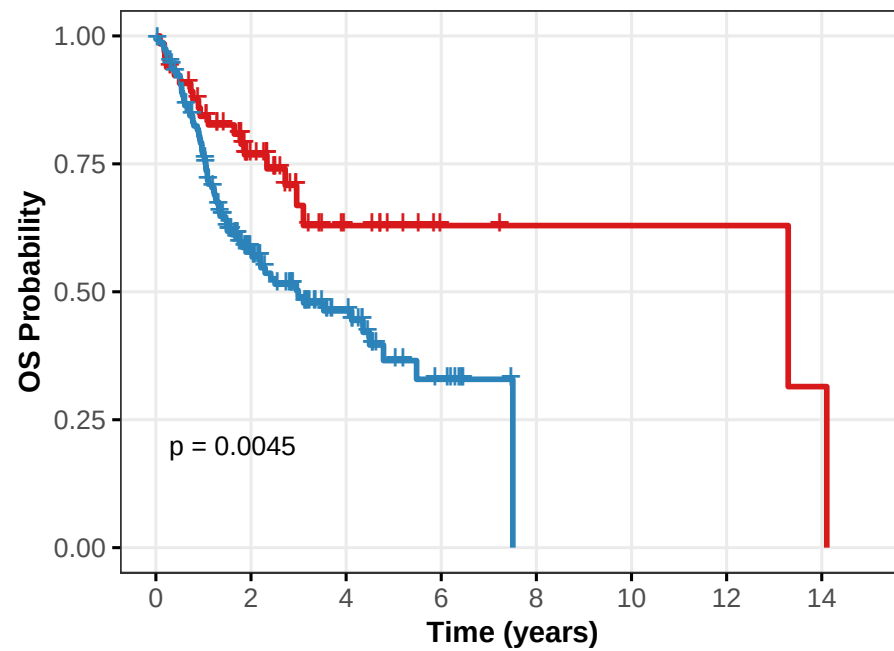
BRCA2
