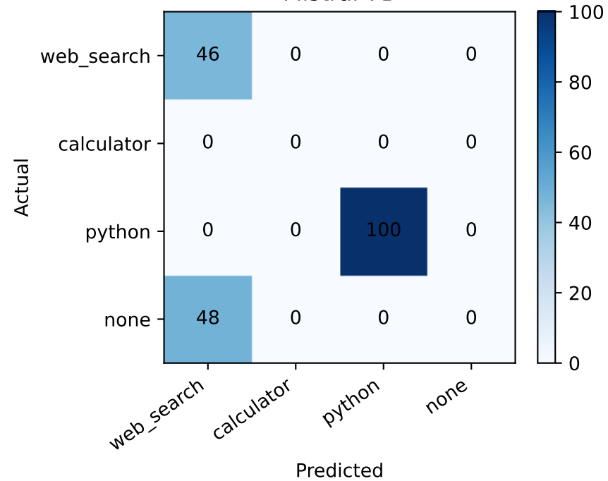
Mistral-7B
