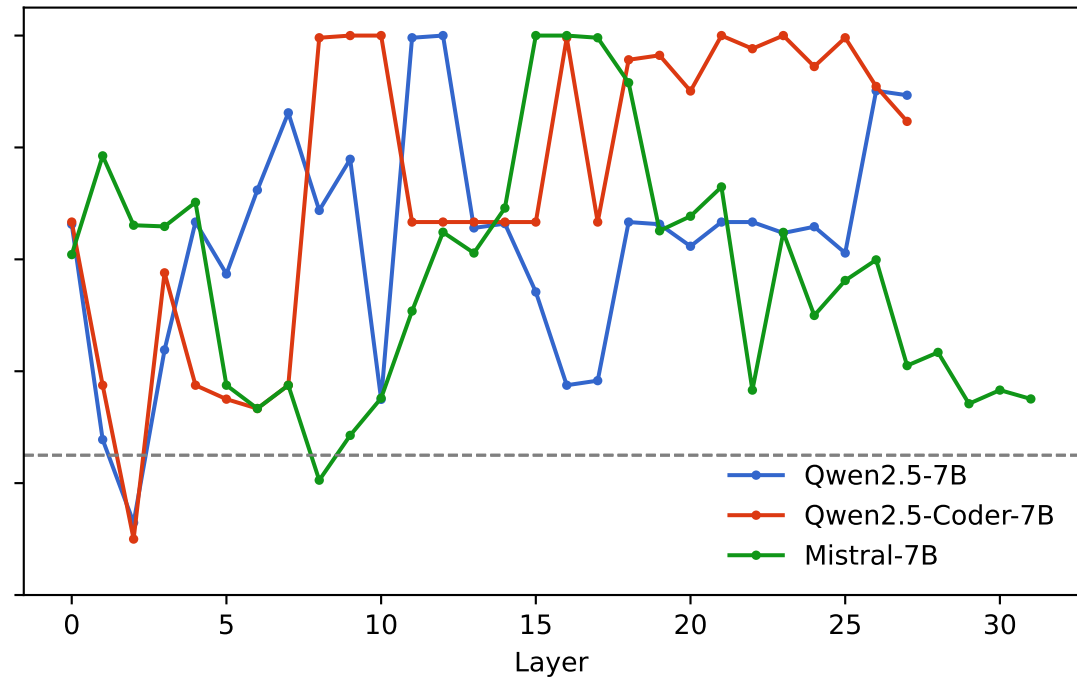
MLP output
