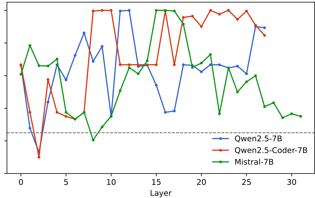
MLP output
