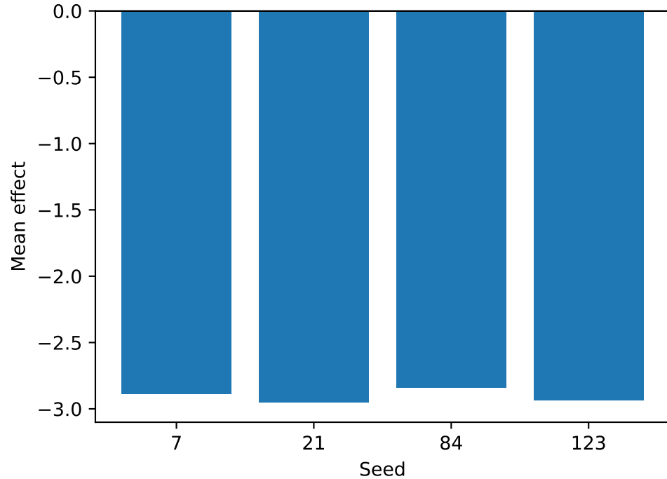
L26H4
