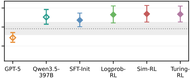
Chat
