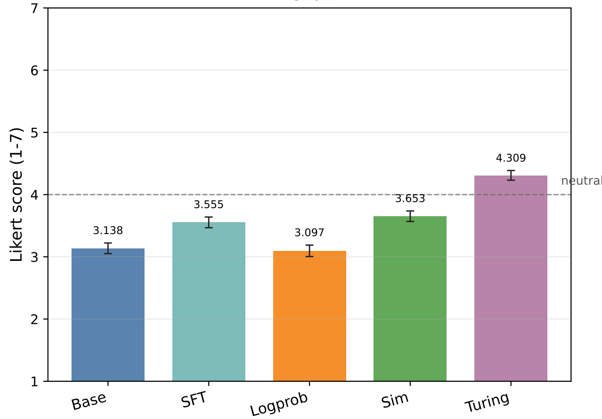
Chat
