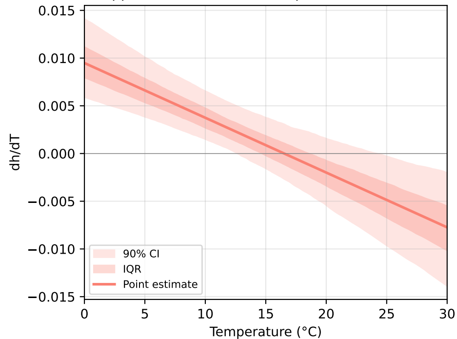
Approach 6e: Actual T component ( h_1 + 2h_2T )
