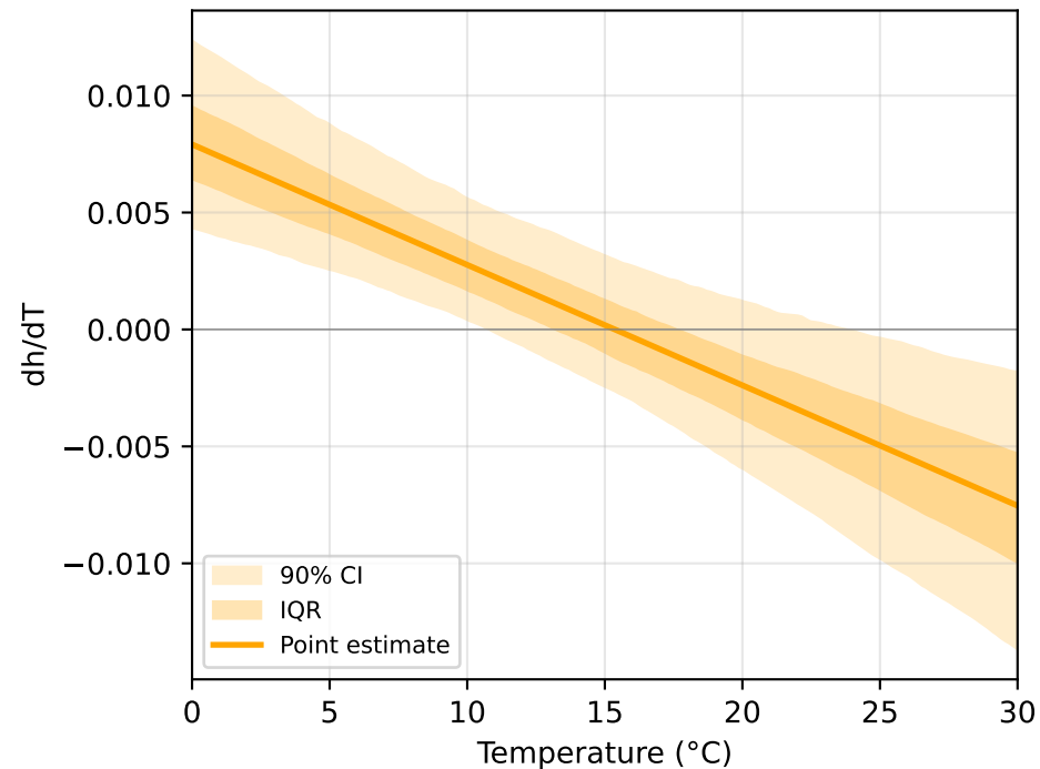
Approach 6e: Actual T component ( h_1 + 2h_2T )
