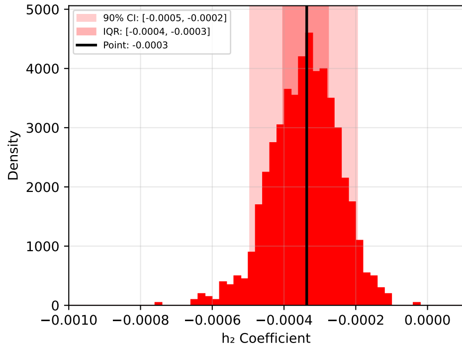
method4: h_2
