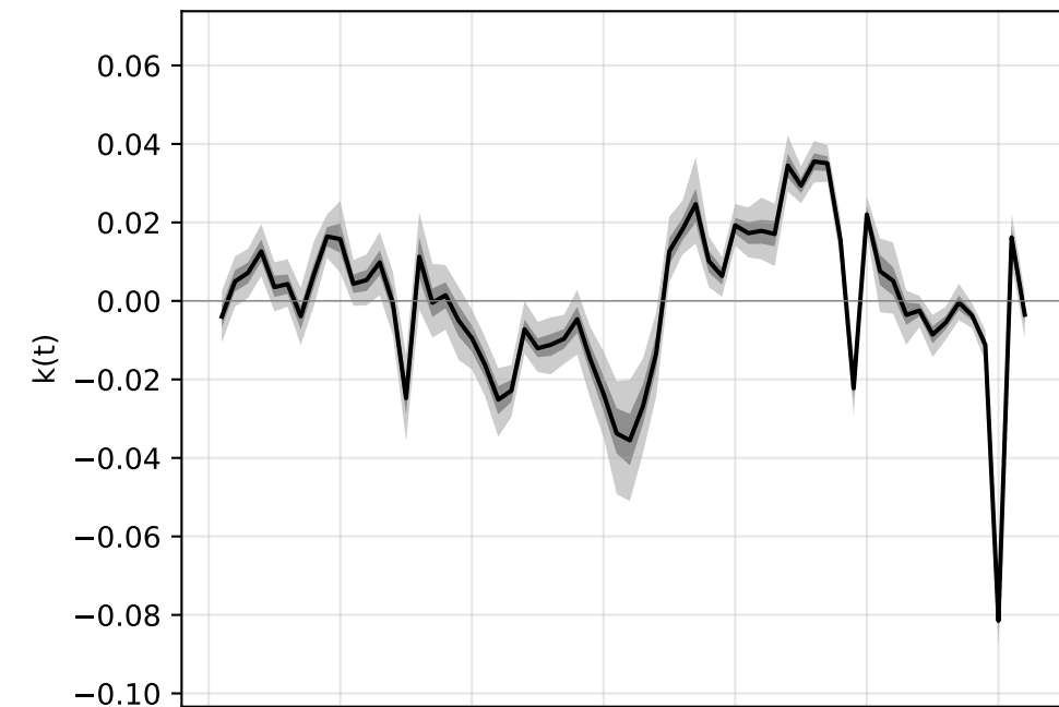
0: Conjoined OLS Fit
