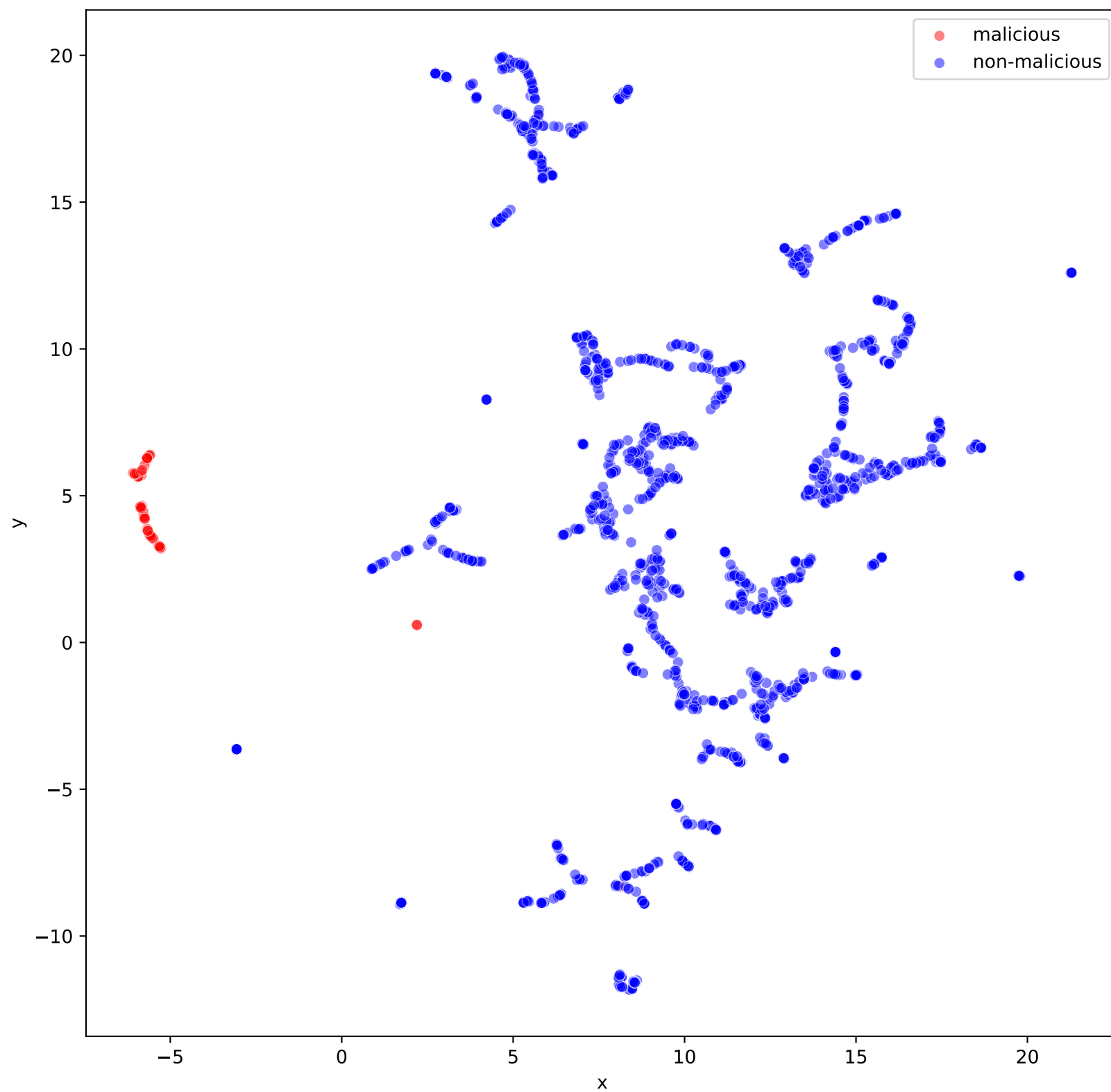
UMAP
