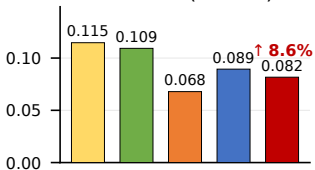
PEMS04 (N=307)
