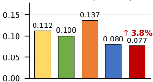
PEMS08 (N=170)
