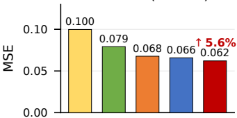
PEMS07 (N=883)
