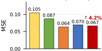
PEMS03 (N=358)
