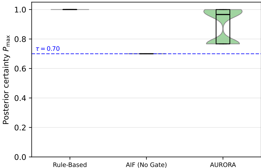
Posterior certainty per agent
