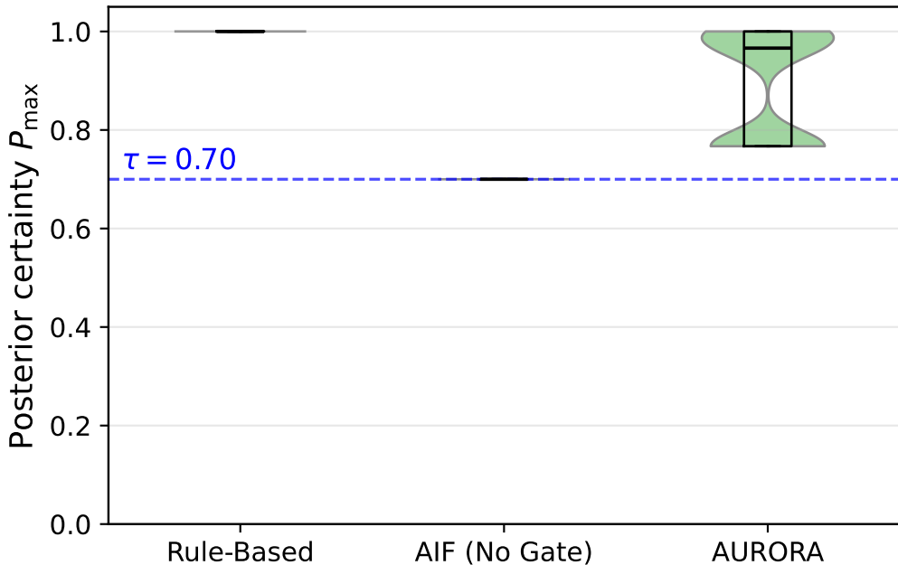
Posterior certainty per agent
