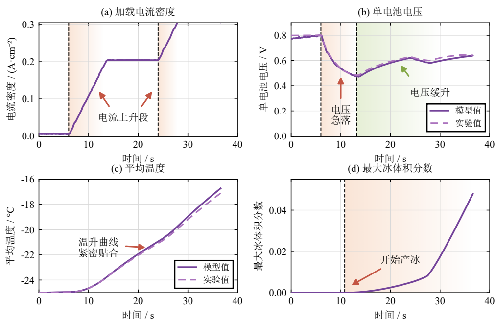
图 4-3 -25^{\circ}C 工况模型与实验对比
