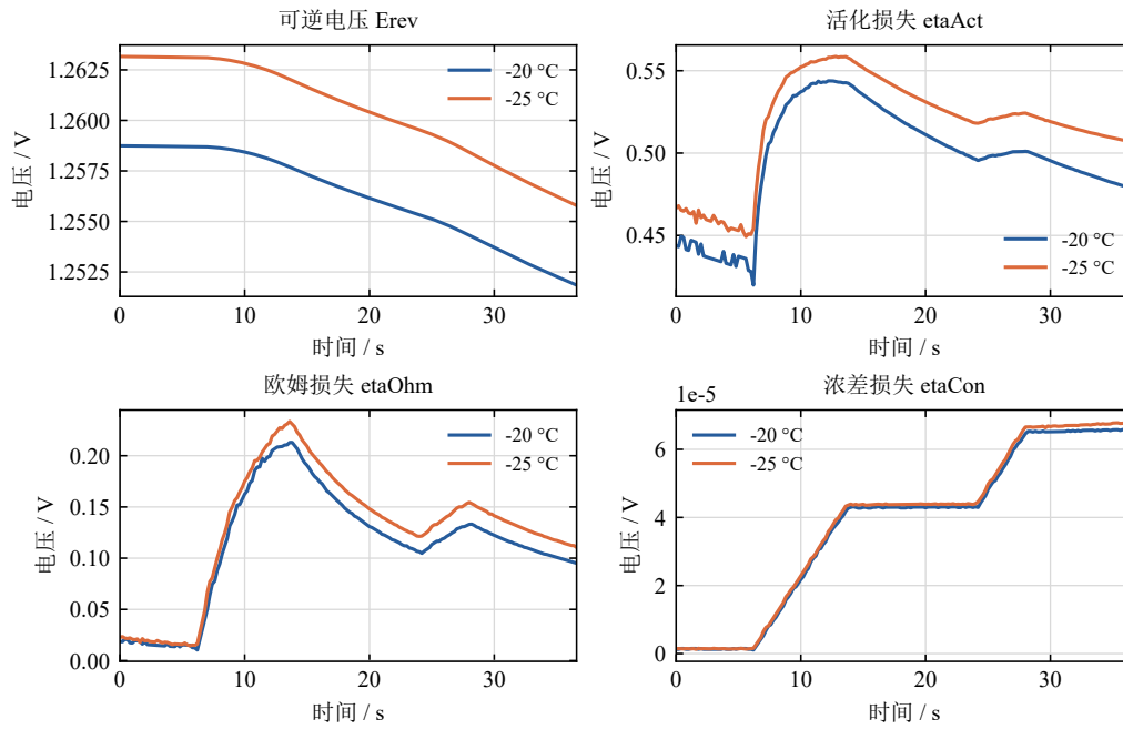
图 4-5 可逆电压与三项极化损失的时间历程
