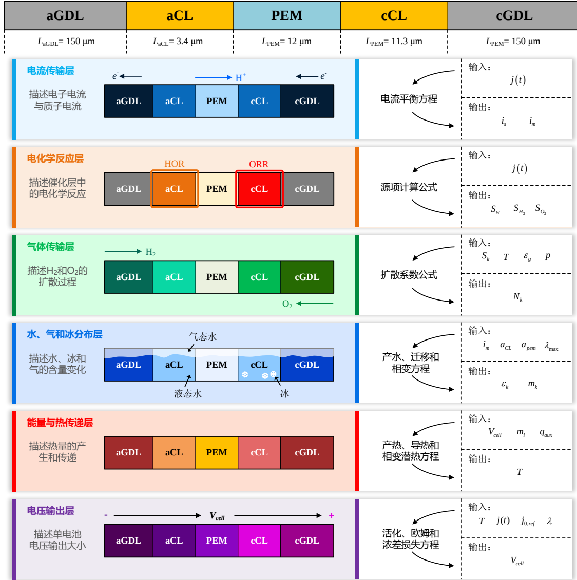
PEM燃料电池一维多状态耦合图
