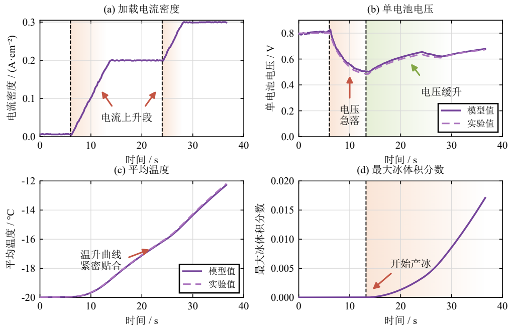
图 4-2 -20 °C 工况模型与实验对比
