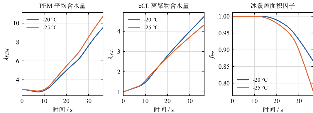
图 4-6 PEM 与 cCL 离子物含水量及水合、冰覆盖面积因子
