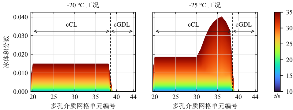
图 4-4 10–35 s 内阴极侧冰体积分数的空间分布与演化
