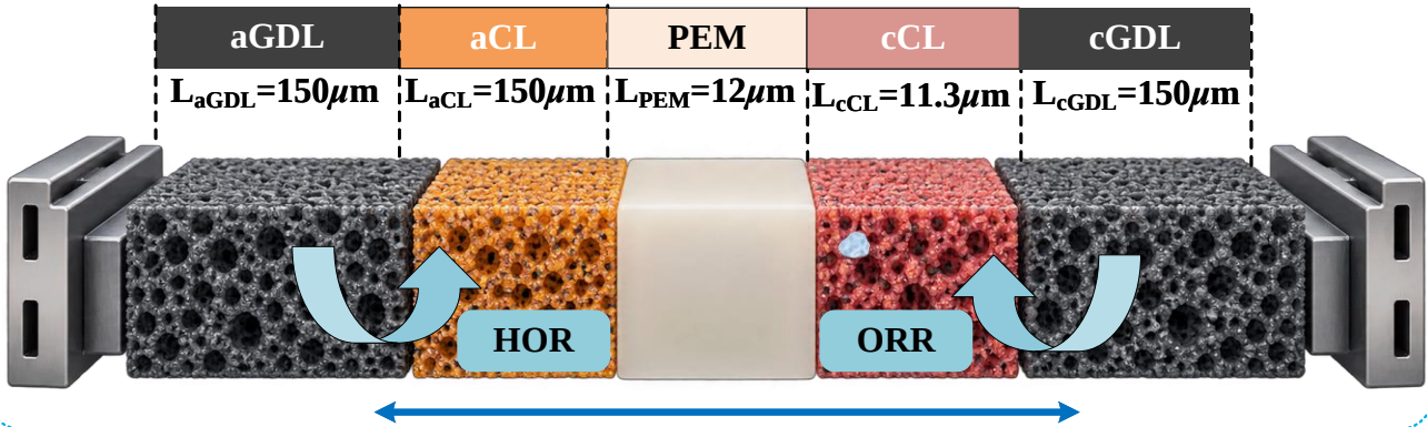
(a)一维质子交换膜燃料电池结构及主要传输过程
