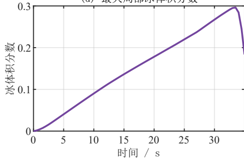
(d) 最大局部冰体积分数
