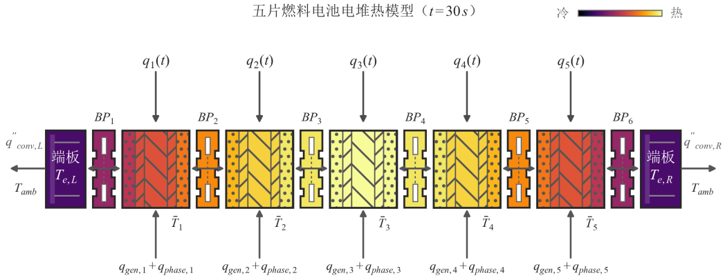
图 6-1 五片电堆辅助加热与热耦合示意（协同加热约 30 s，双极板色彩按相邻求解节点插值）
