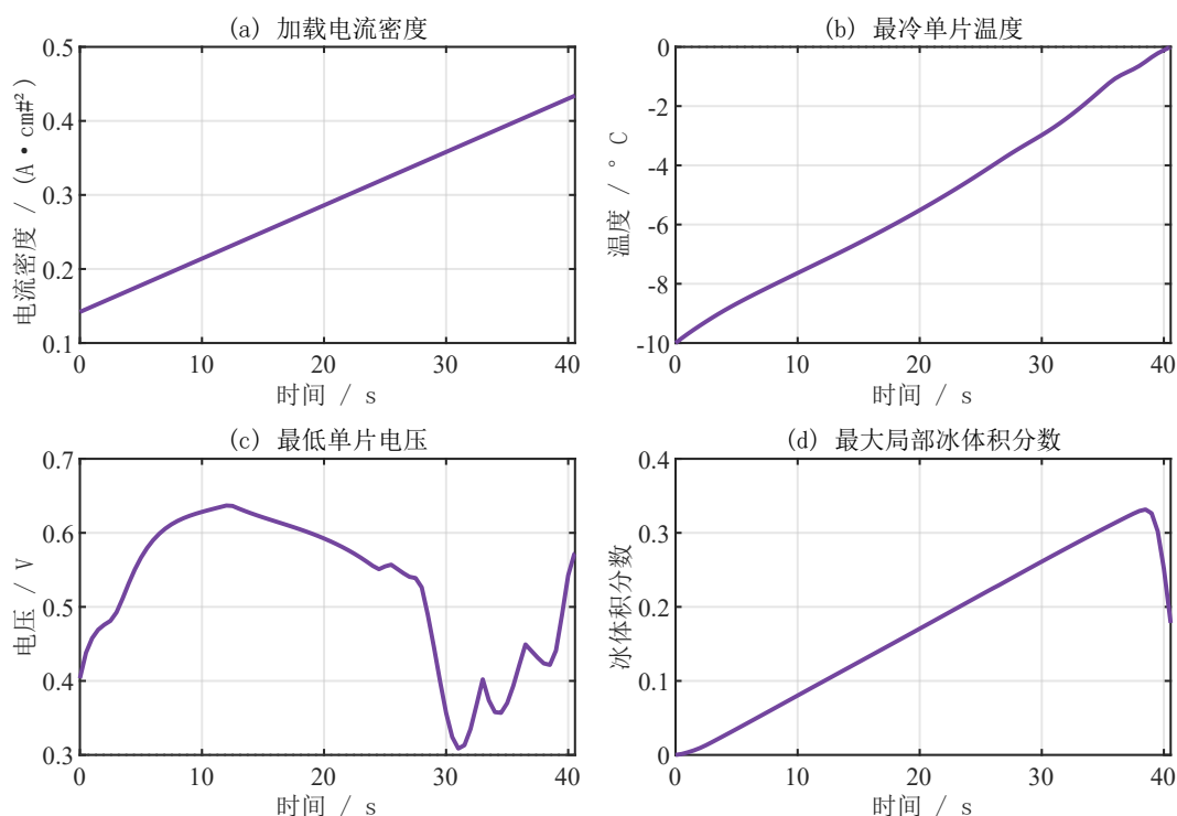
图 5-5 选定线性升载曲线的电流、温度、电压与冰量
