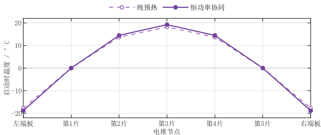
图 6-4 两种策略各自启动完成时的端板与五片单电池平均温度
