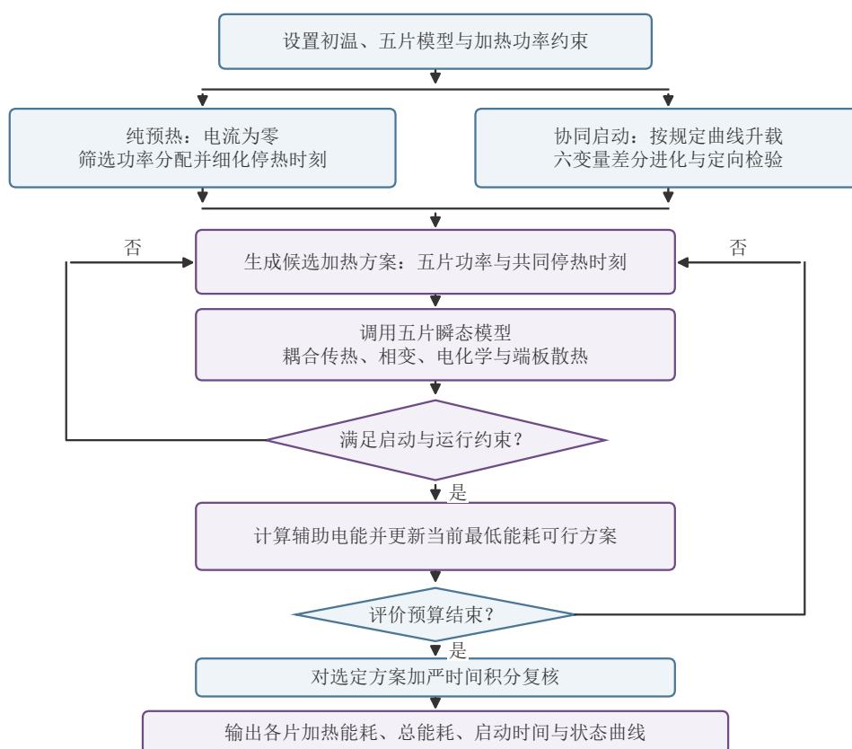
图 6-2 问题三两种辅助加热策略的参数搜索与仿真评价流程
