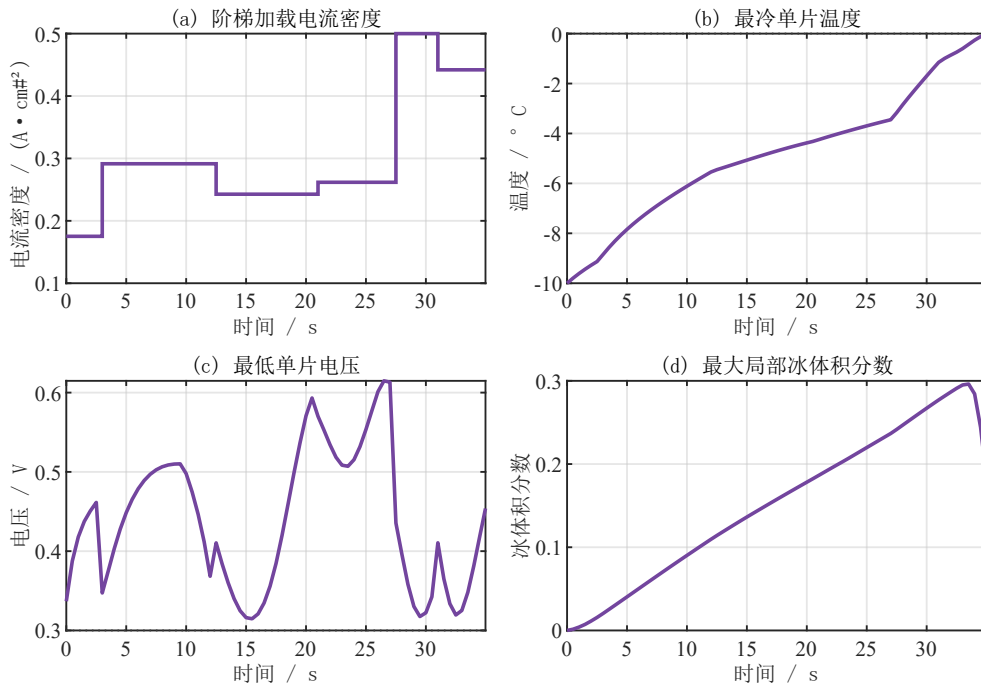
图 5-6 选定阶梯加载曲线在 -10\text{ }^{\circ}\text{C} 下的电流、温度、电压与冰量
