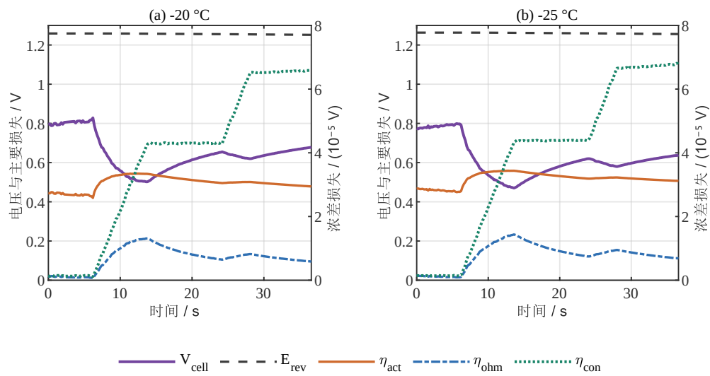
图 4-5 两个低温工况的单电池电压、可逆电压与三项极化损失
