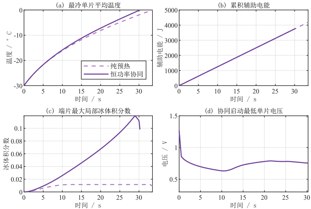
图 6-3 辅助冷启动过程的温度、能耗、端片冰量及电压
