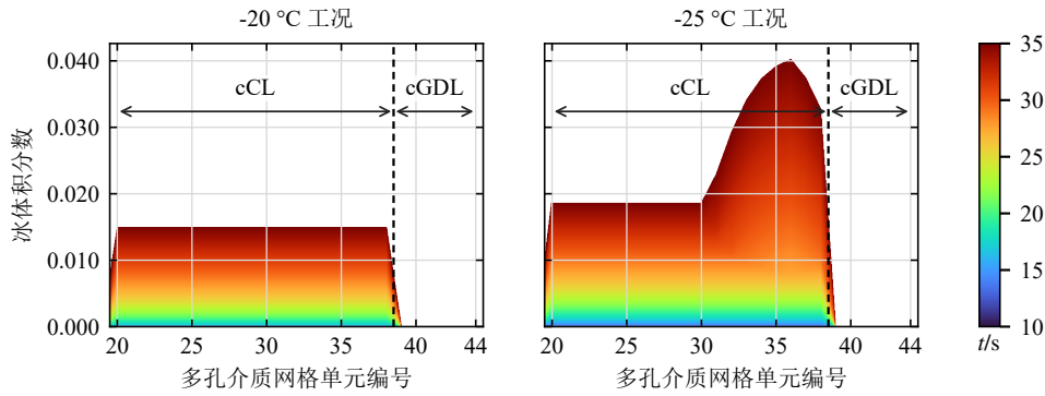
图 4-4 10–35 s 内阴极侧冰体积分数的空间分布与演化
