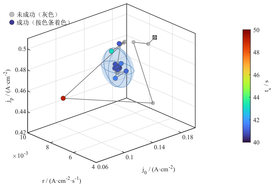
图 5-4 线性升载代理模型选点的空间轨迹与末期搜索邻域（灰色点为未成功评价）
