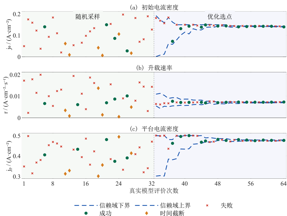
图 5-3 线性升载参数的搜索过程
