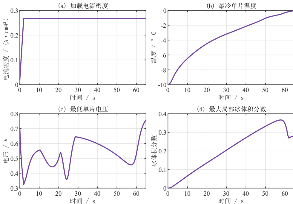
图 5-2 选定恒流加载曲线的电流、温度、电压与最大冰体积分数
