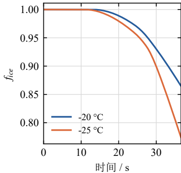
冰覆盖面积因子
