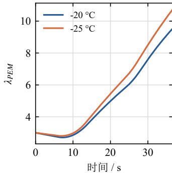
PEM 平均含水量
