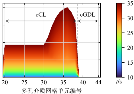
-25 °C 工况
