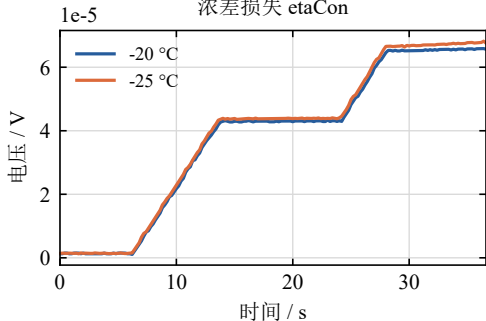
浓差损失 \eta_{con}
