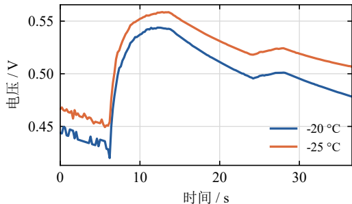
浓差损失 \eta_{con}
