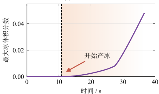
(d) 最大冰体积分数
