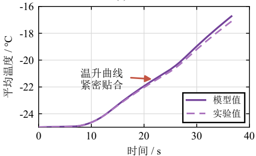
(c) 平均温度
