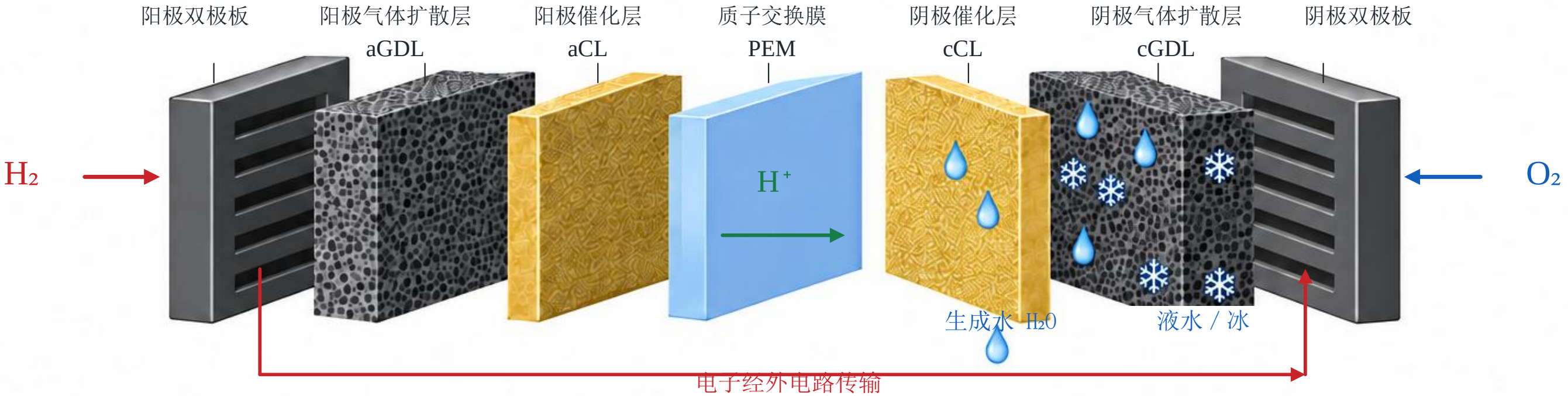
(a) 单电池分层结构
