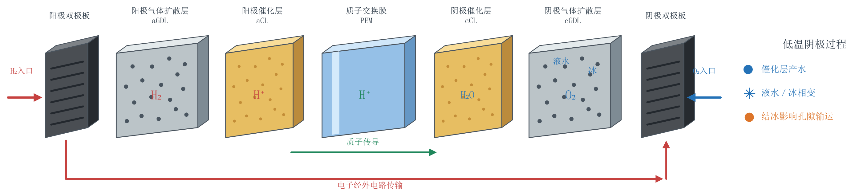
(b) 一维求解区域（沿厚度 x 方向）
