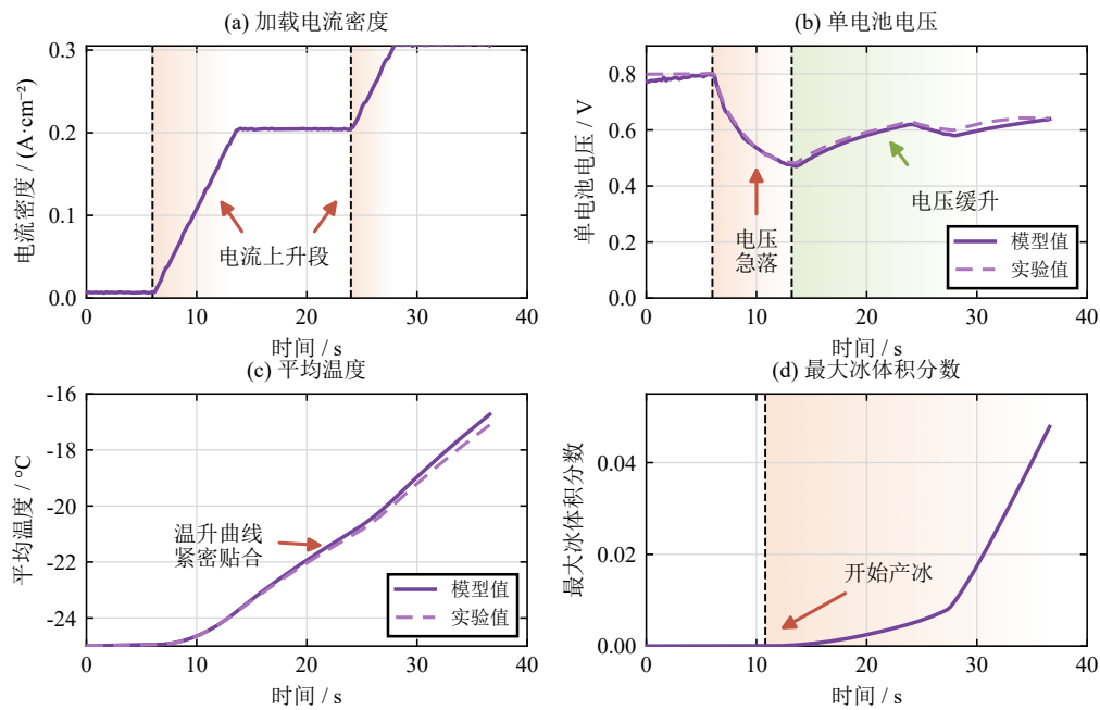
图 4-2 -25^{\circ}C 工况模型与实验对比
