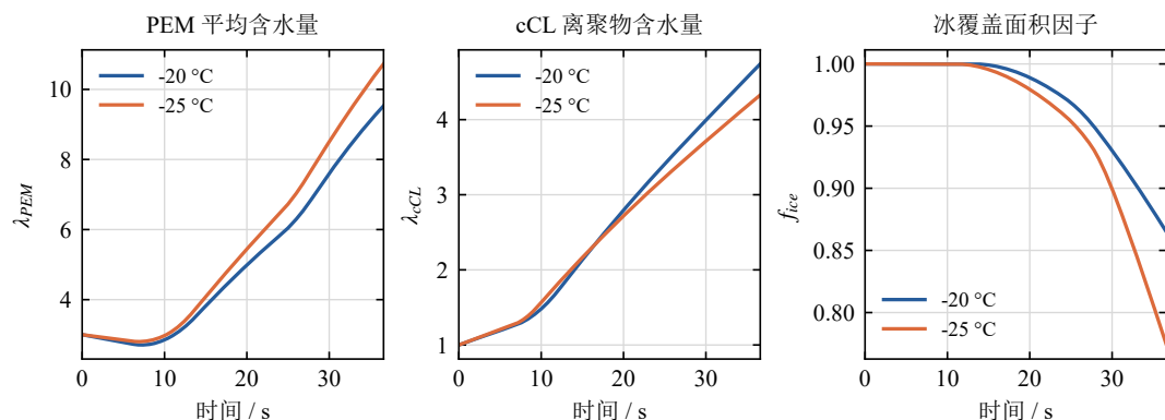
图 4-5 PEM 与 cCL 离聚物含水量及水合、冰覆盖面积因子
