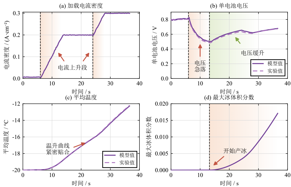
图 4-1 -20 ^{\circ}\text{C} 工况模型与实验对比
