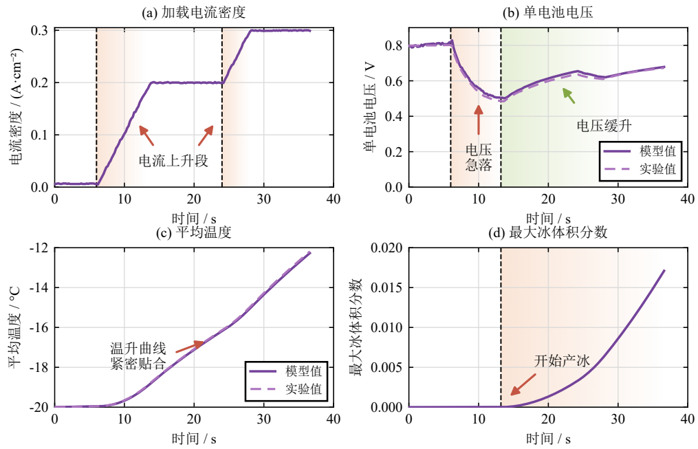
图 4-1 -20^{\circ}C 工况模型与实验对比
