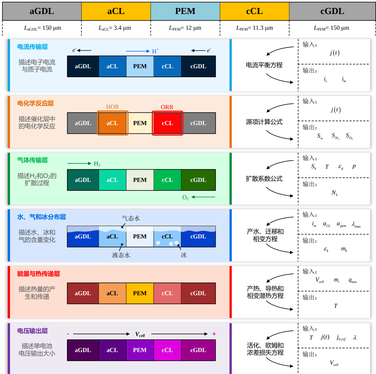
PEM燃料电池一维多状态耦合图
