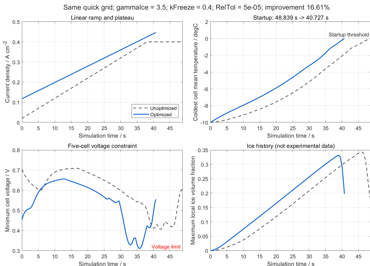
图 5-1 未优化与优化线性加载方案在同一快速网格下的模型仿真对比
