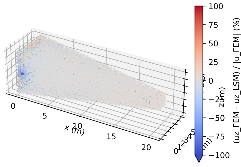
Error in z (max |\cdot| = 348.22 %)
