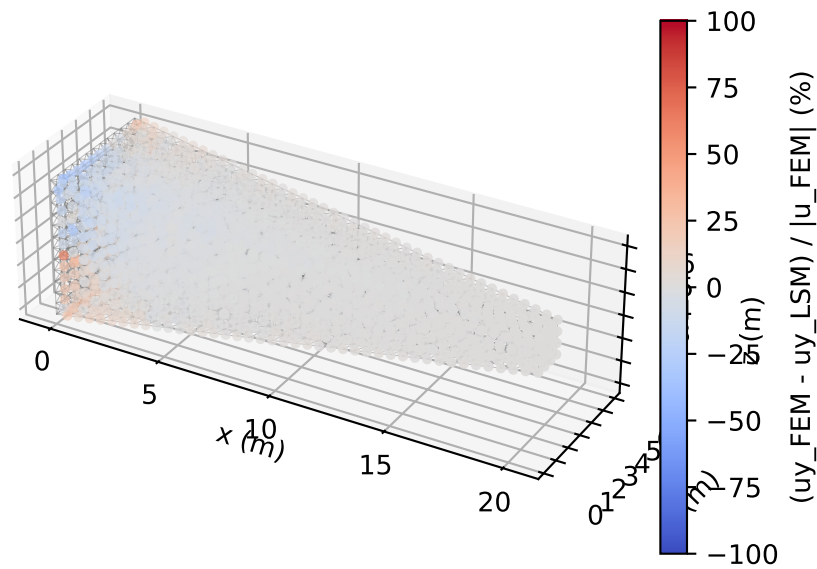
Error in y (max |\cdot| = 57.05 %)
