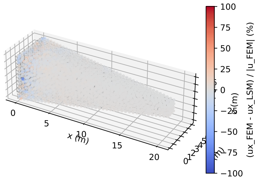
Error in x (max |\cdot| = 69.28 %)
