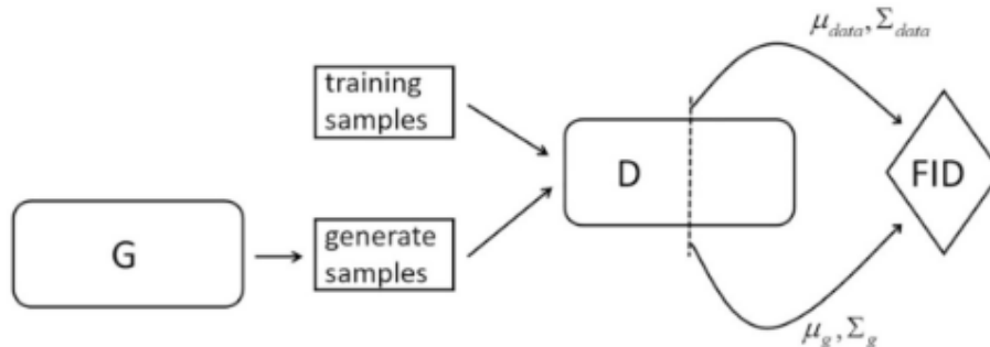
Abb. 6.1: Darstellung der FID-Berechnung [49, S. 130]
