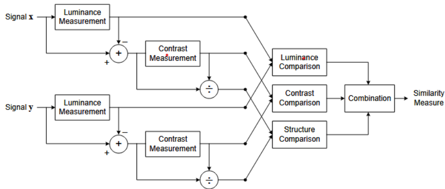
Abb. 6.2: Darstellung der SSIM-Berechnung [69, S. 5]
