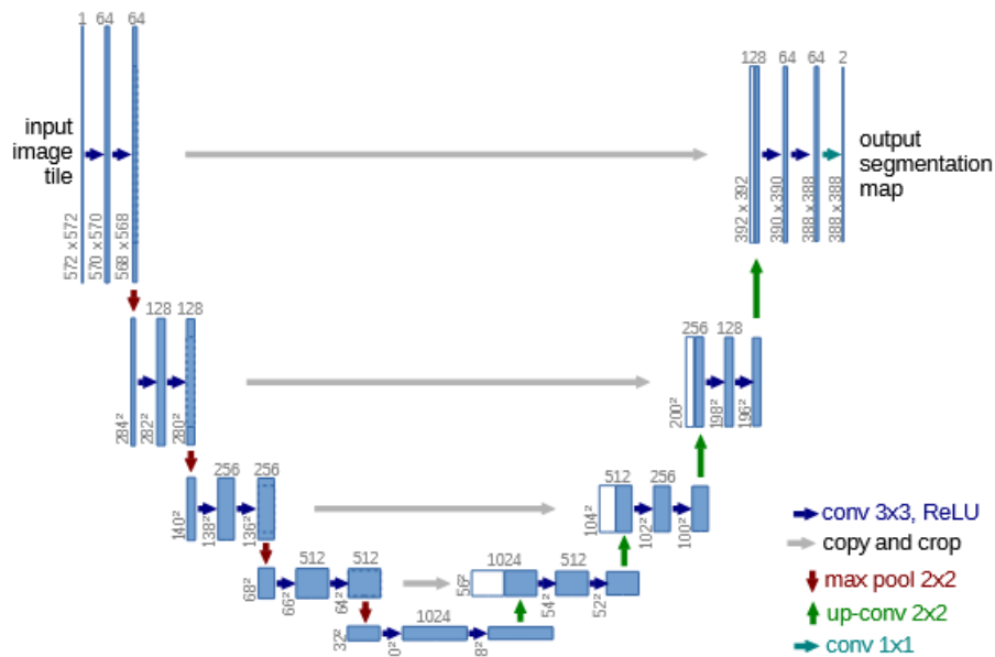
Abb. 5.5: U-Net Architektur [49, S. 2]
