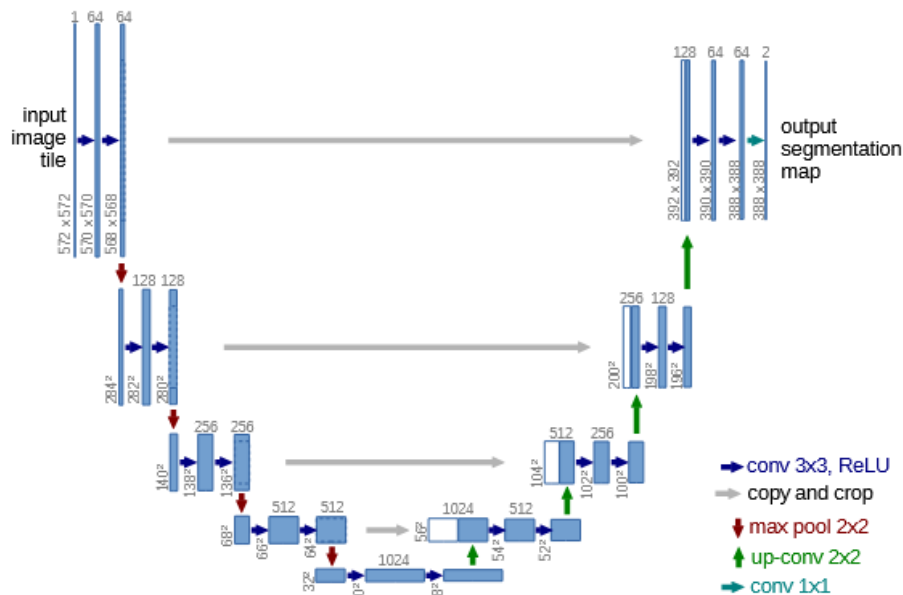
Abb. 5.5: U-Net Architektur [52, S. 2]
