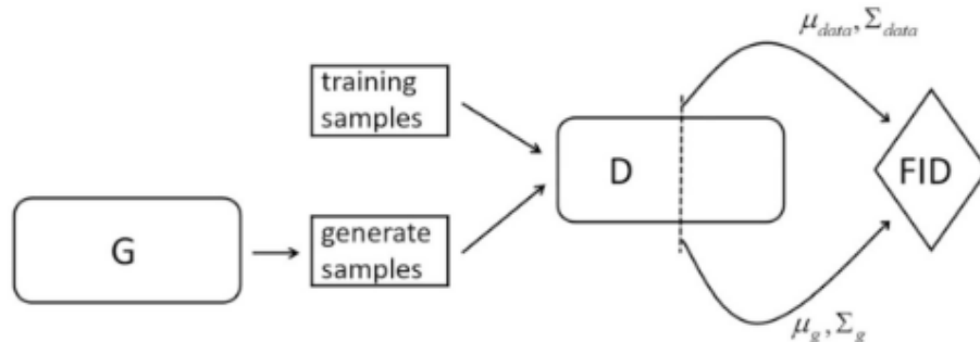
Abb. 6.1: Darstellung der FID-Berechnung [64, S. 130]
