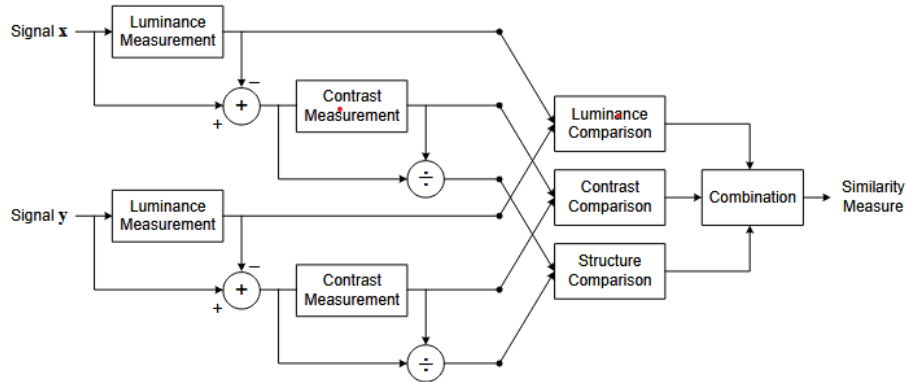
Abb. 6.2: Darstellung der SSIM-Berechnung [52, S. 5]
