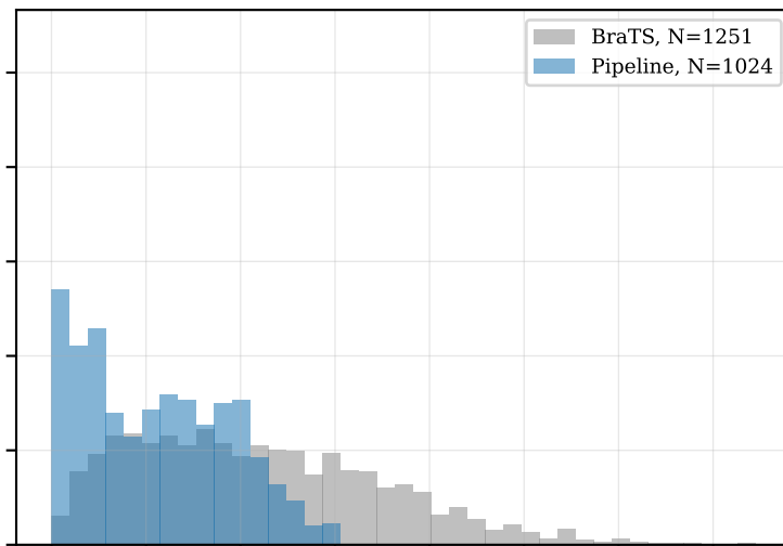
DDIM (50)
