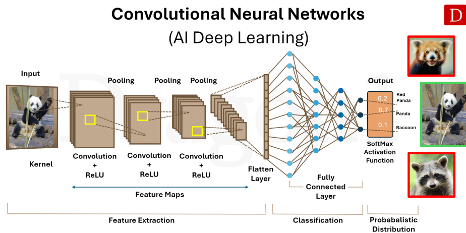
Abb. 5.4: CNN
