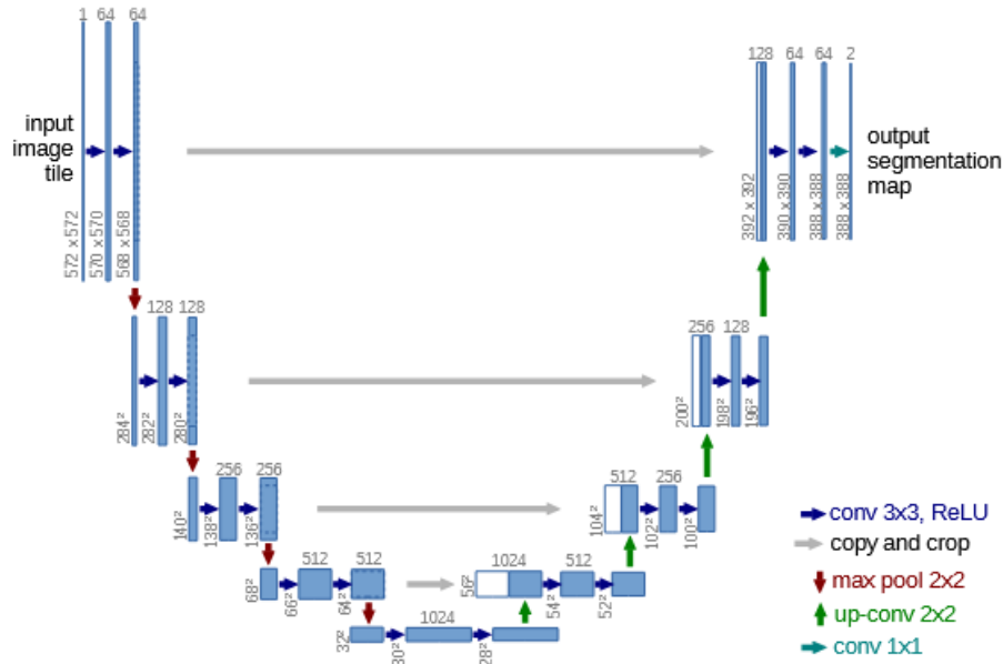
Abb. 5.5: U-Net Architektur [51, S. 2]
