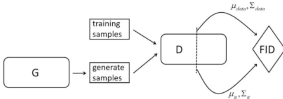
Abb. 6.1: Darstellung der FID-Berechnung [68, S. 130]
