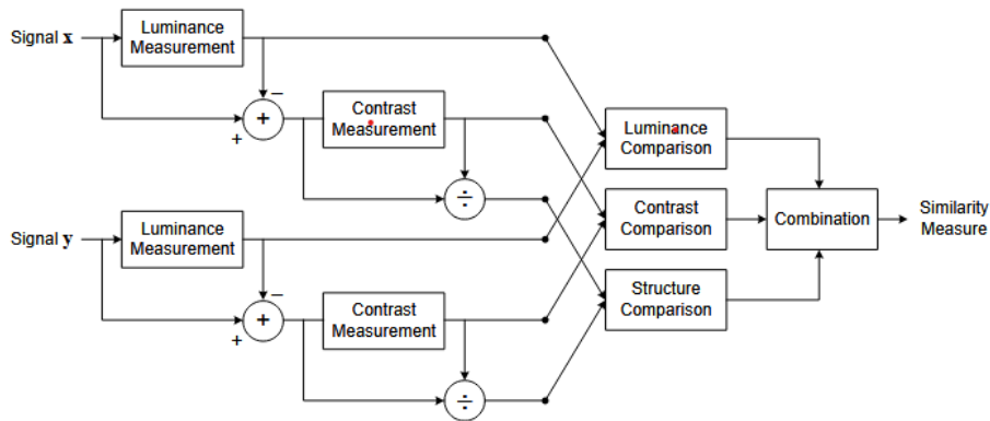
Abb. 6.2: Darstellung der SSIM-Berechnung [65, S. 5]
