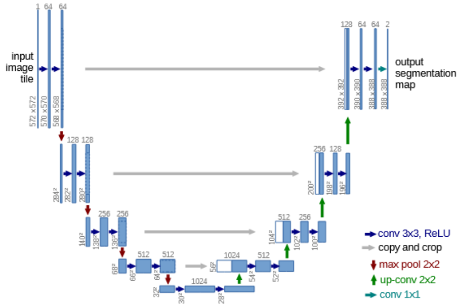
Abb. 5.5: U-Net Architektur [34, S. 2]
