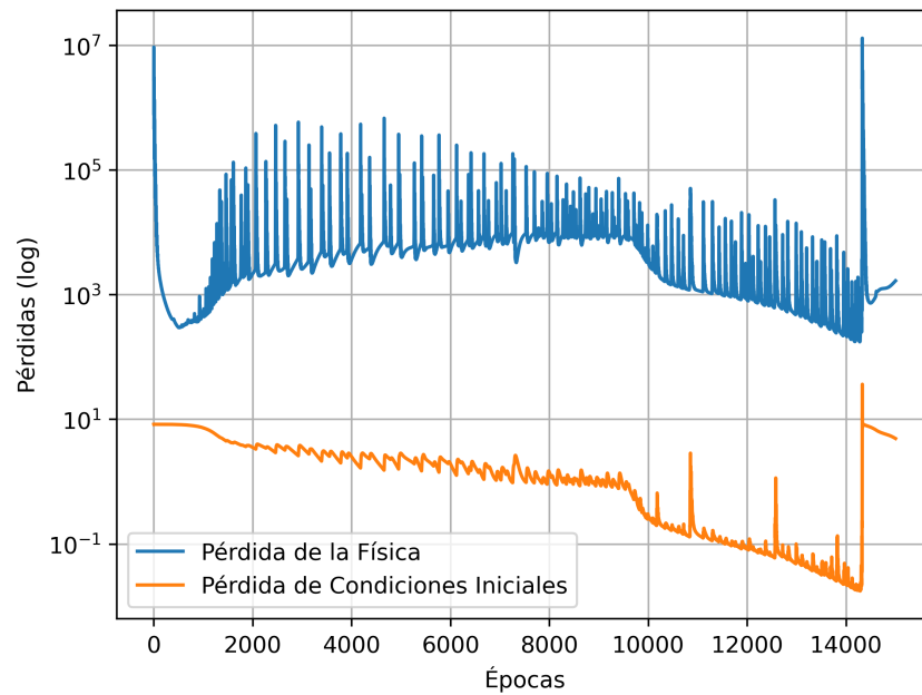
Figura 3: Loss vs Epochs para arquitectura inicial sin Scheduler. Notamos oscilación en la perdida para números altos de epochs
