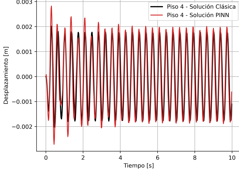
Figura 15: Resultado para 40 piso de red SIREN usando optimizador SOAP sobre 10 segundos con \omega_{fuerza} = 2.75 Hz.
