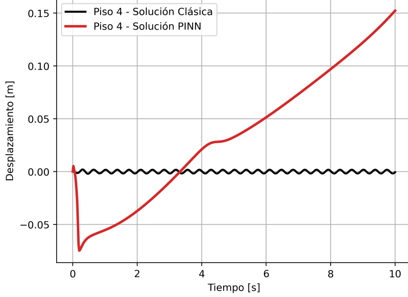
Figura 6: Resultado de modelo Tanh para el 4º piso sobre 10 segundos con \omega_{fuerza} = 2.75 Hz. Este gráfico es representativo de la tendencia en el resto de los pisos.
