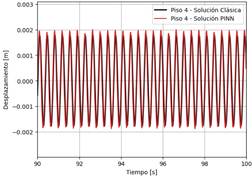
Figura 18: Solución de la red gráfícada para intervalo [90;100] segundos para 4o piso con \omega_{fuerza} = 2,75 Hertz.
