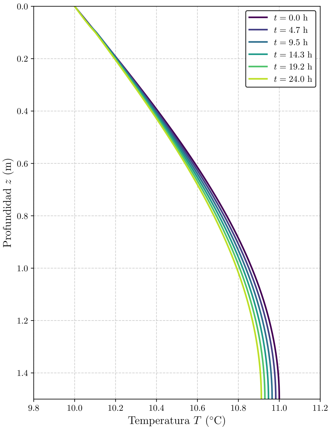
Evolución del perfil de temperatura T(z, t) a x = 0.5 m
