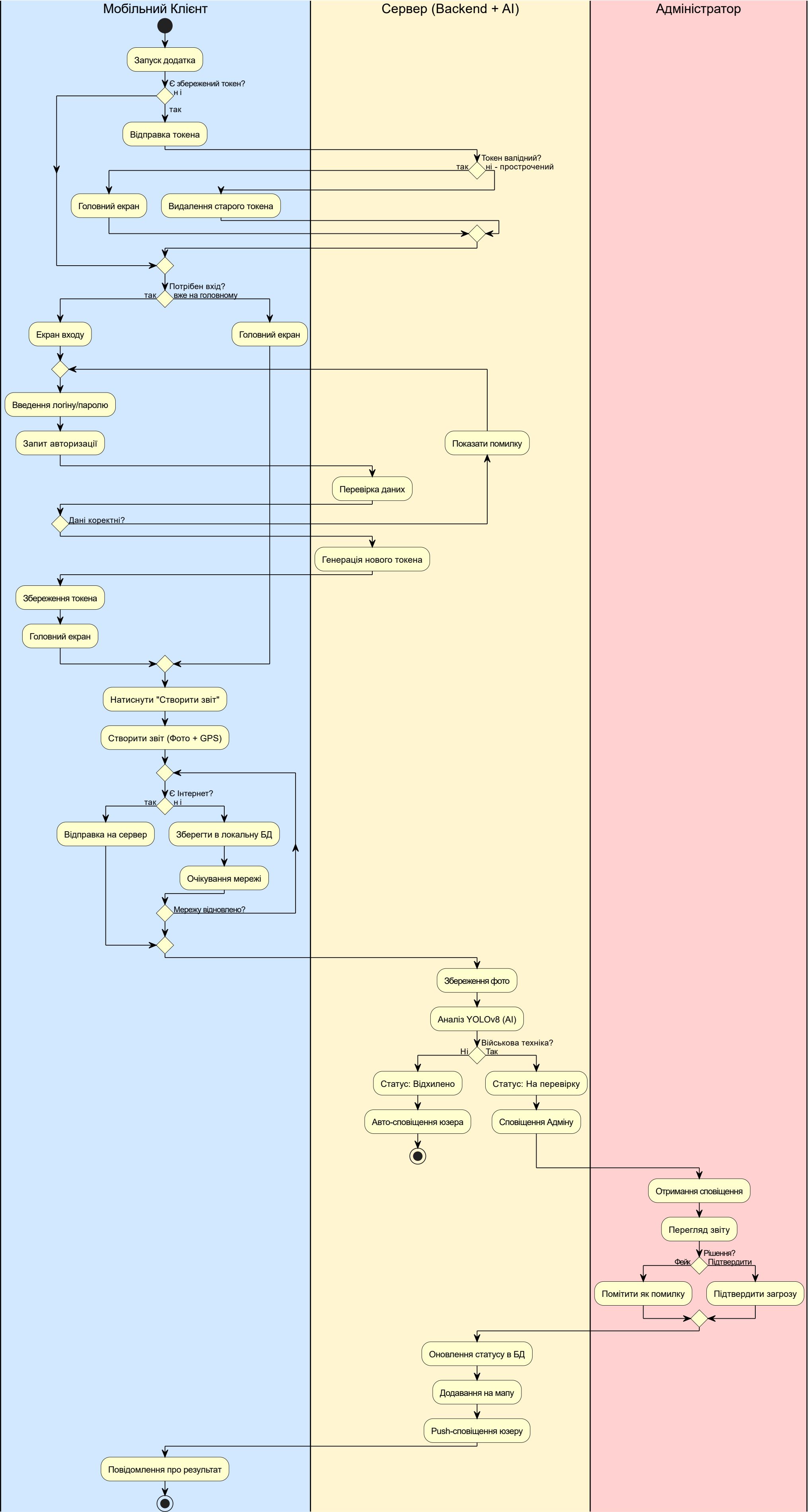
Діаграма діяльності "Системи автоматичного розпізнавання військової техніки та інфраструктури за допомогою технологій ШІ"
