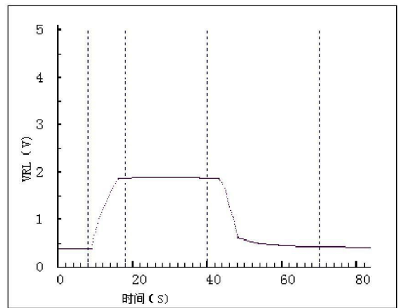
图 6 响应恢复特性
