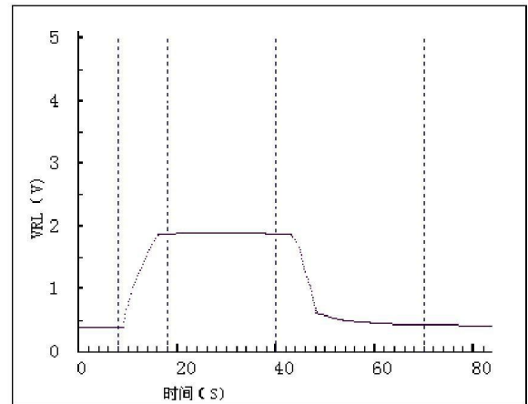
图 6 响应恢复特性
