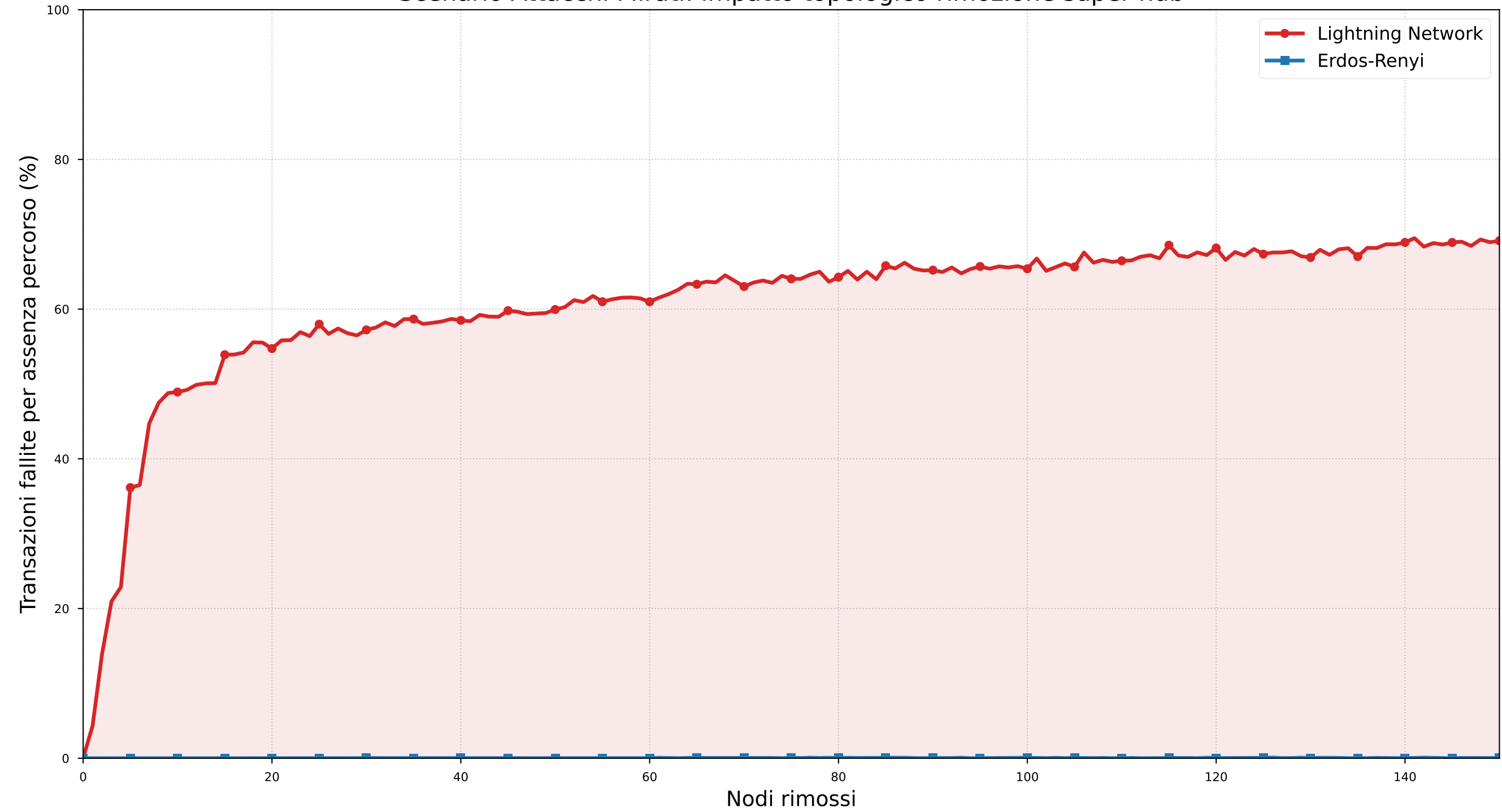
Scenario Attacchi Mirati: impatto topologico rimozione super hub
