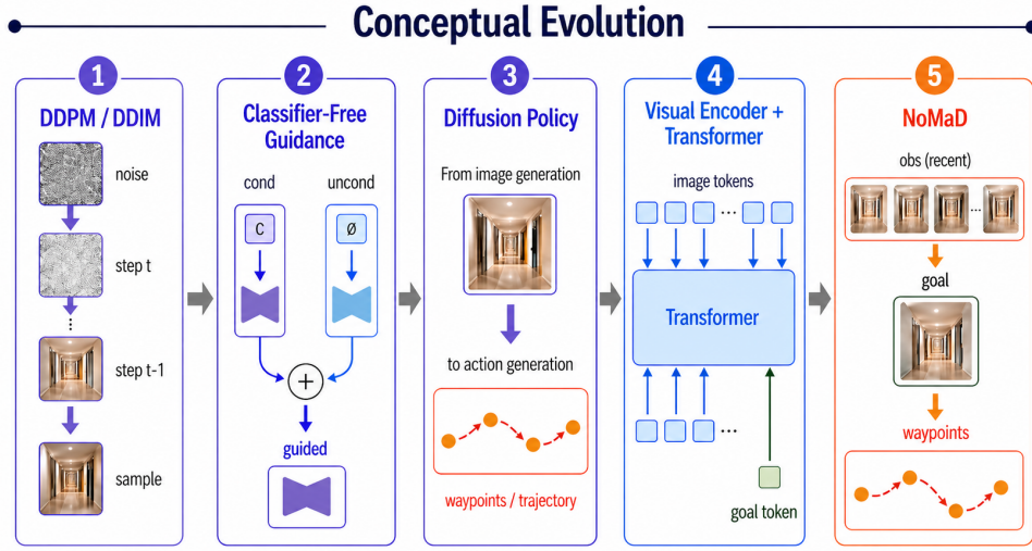
图 2.3 扩散模型、扩散策略、ViT 编码器与 NoMaD 系统之间的技术演化关系。从左到右依次为基础扩散理论（DDPM/DDIM）、条件引导方法（CFG）、扩散策略（Diffusion Policy）以及 NoMaD 的架构
