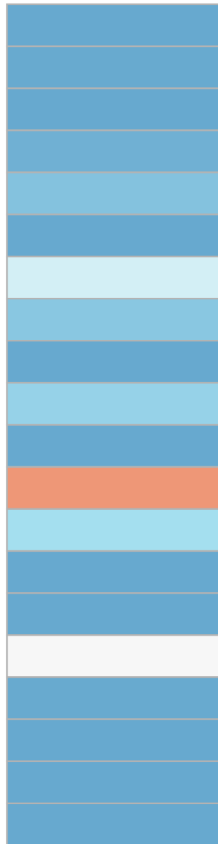
MalReBay
