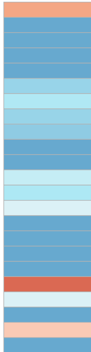
MalReBay
