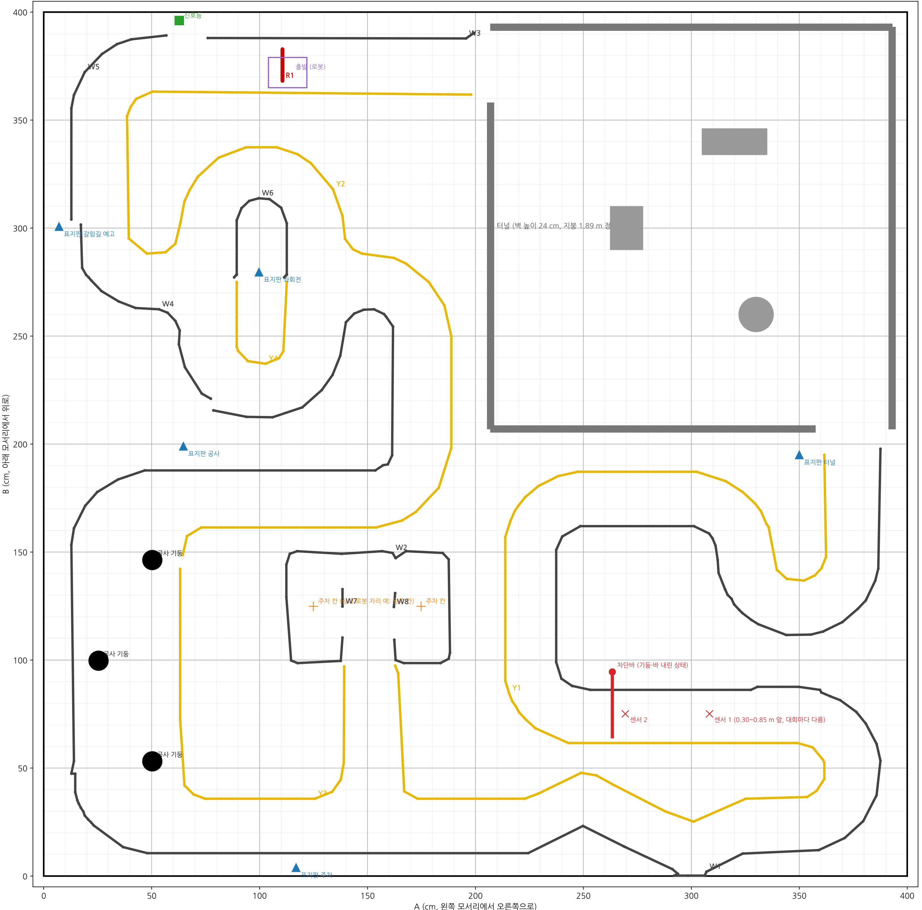
오토레이스 연습 경기장 테이프 도면 — 4 m × 4 m, 선 중심선 기준 (cm)
