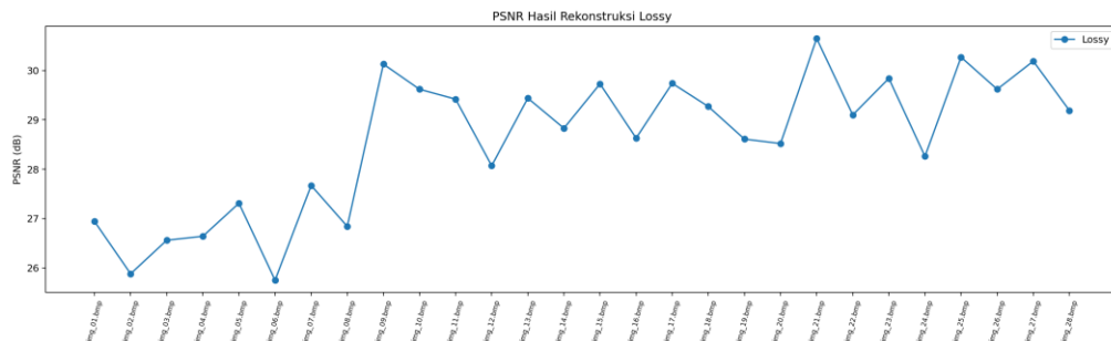
Gambar 4. Grafik PSNR hasil rekonstruksi lossy pada 28 gambar.
