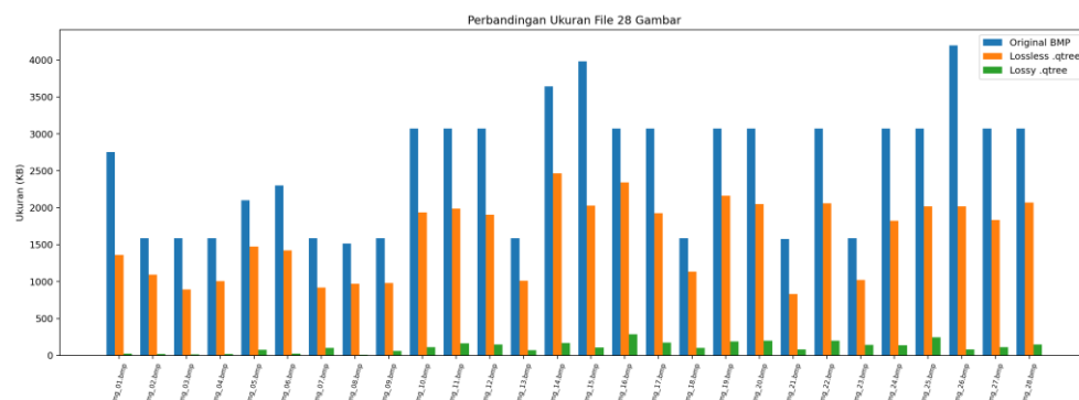
Gambar 1. Grafik perbandingan ukuran file asli dan hasil kompresi.
