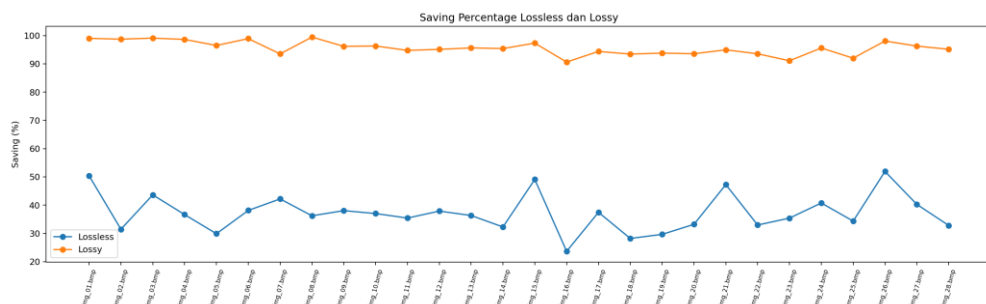
Gambar 3. Grafik saving percentage lossless dan lossy pada 28 gambar.
