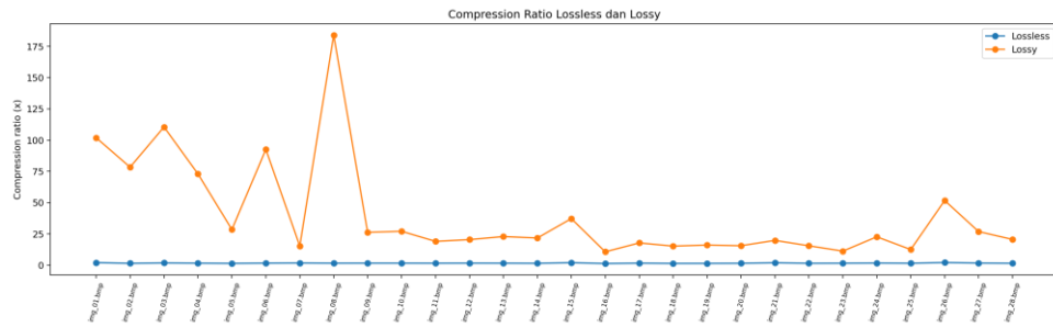
Gambar 2. Grafik compression ratio lossless dan lossy pada 28 gambar.
