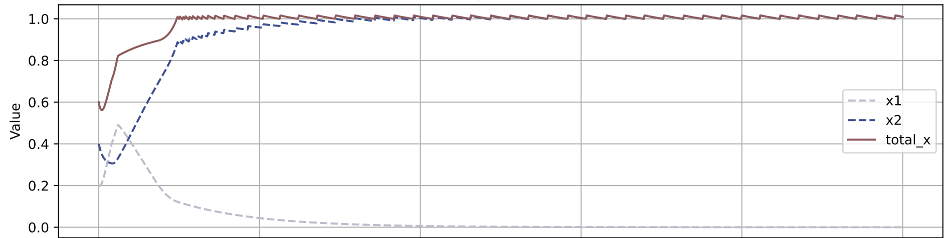
Trajectories
